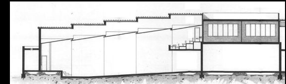
SECCION A-B
